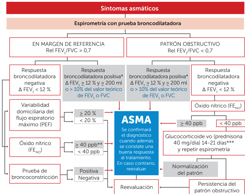
FIGURA 2.1. Algoritmo diagnóstico.
